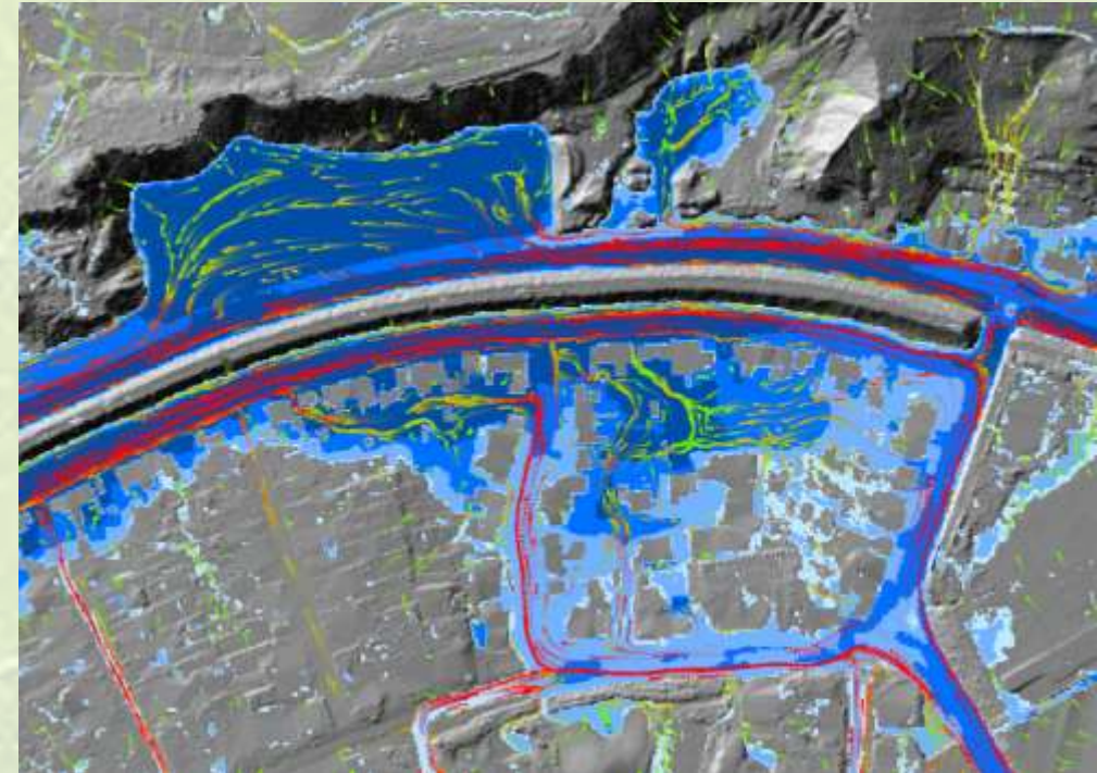
Auszug Starkregengefahrenkarte: Extremes Starkregenereignis mit Schummerung, HRB Übach
